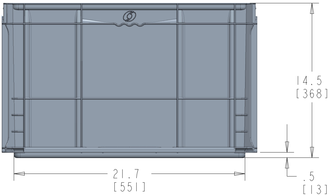
LONG SIDE
