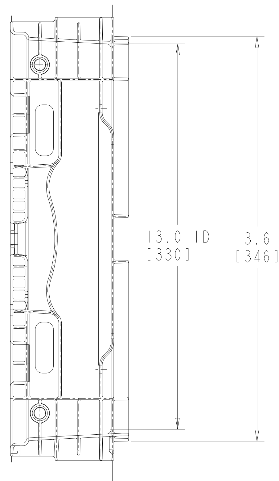
LONG SIDE
