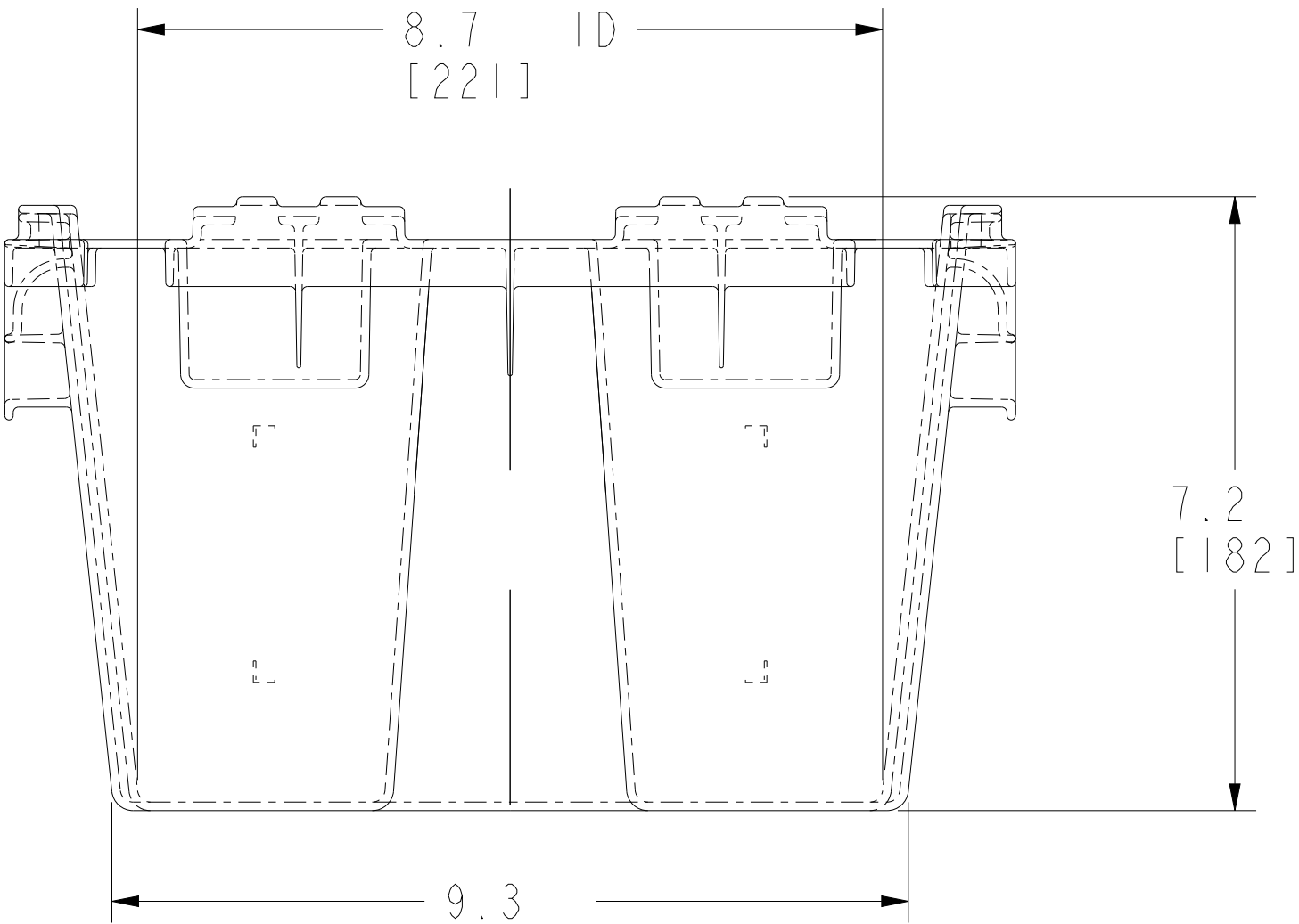
LONG SIDE
