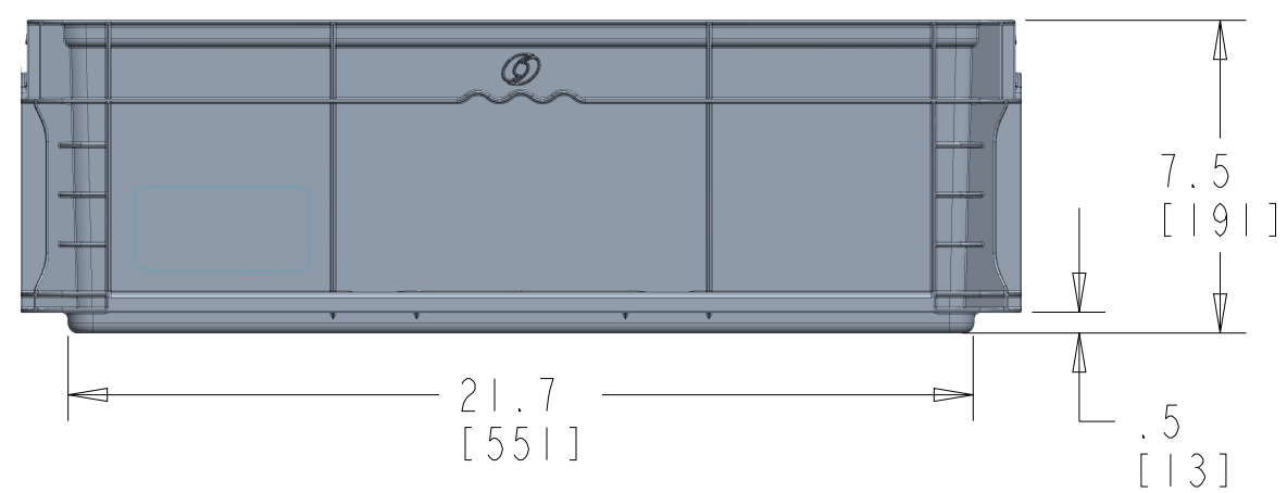
LONG SIDE
